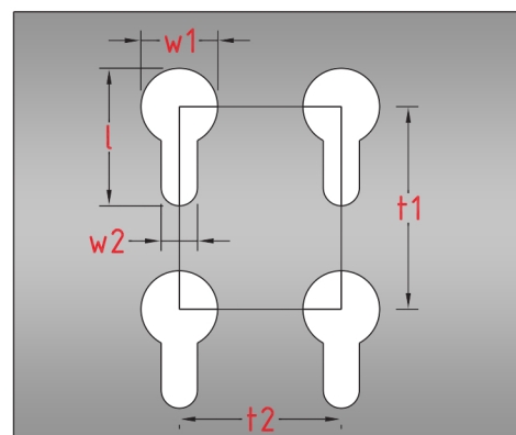
OZNAKA PERFORACIJE: K (w•l) U (t1•t2)
