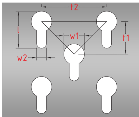
OZNAKA PERFORACIJE: K (w•l) Z (t1•t2)
