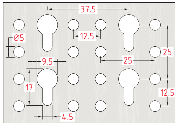
Perforacija: Okrugli ključ otvor Oznaka: K (9,5 • 17) R (5)
