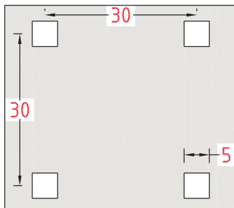
Oznaka perforacije: C5 U30
