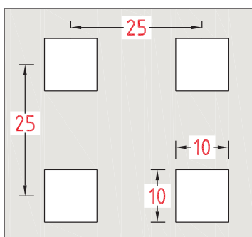
Oznaka perforacije: C10 U25
