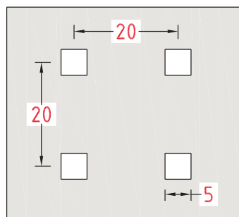
Oznaka perforacije: C5 U20
