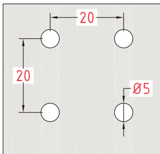
Oznaka perforacije: R5 U20
