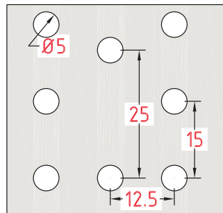
Europorforacija Oznaka: R5 Euro
