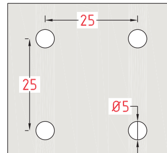
Oznaka perforacije: R5 U25
