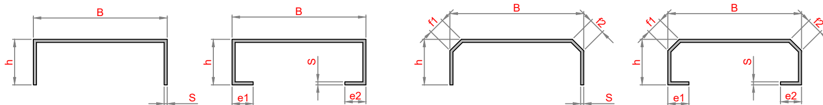
Primeri: Standardno savijanje profila
